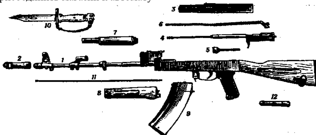
Рис. 9. Основные части и механизмы автомата и его принадлежности:
